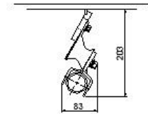
TUNGSTEN CARBIDE MINE DUTY MDX V-TIP
